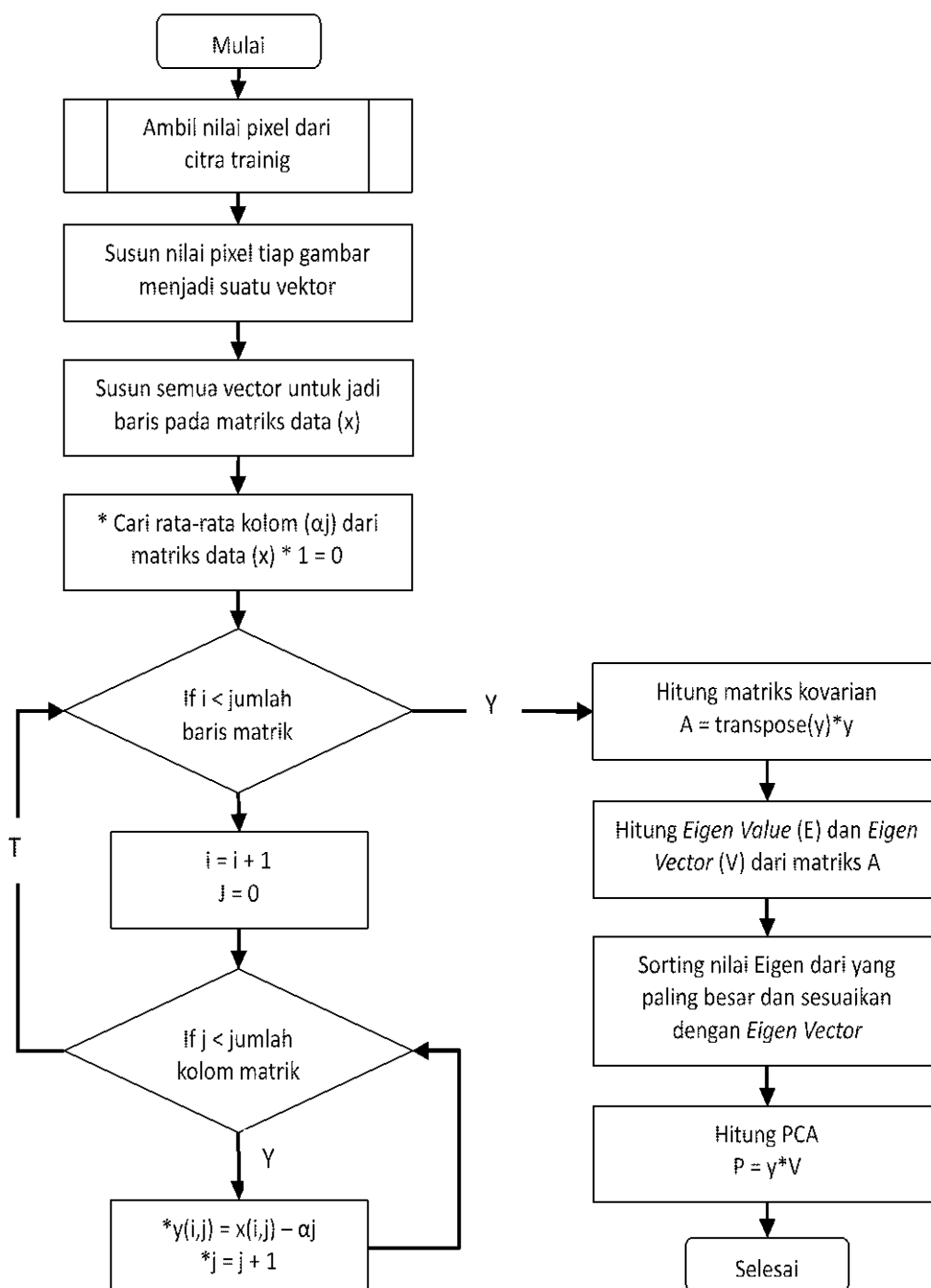
Gambar. 2. Tahapan proses ekstraksi ciri dengan menggunakan PCA
