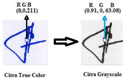
Gambar 9. Perubahan citra true color menjadi grayscale
