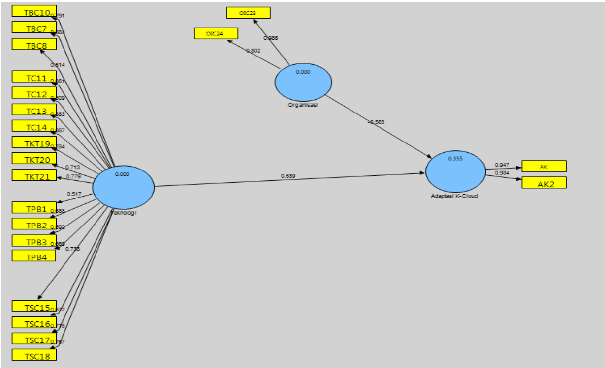
Gambar 2 Model Akhir
